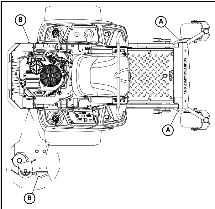
A. Tie-down point—Front | B. Tie-down point—Rear
